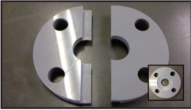
割フランジ 25A
